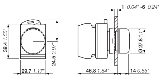
Dimensioni (mm, pollici)
