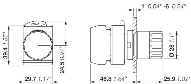
BMD.. Dimensioni (mm, pollici)
